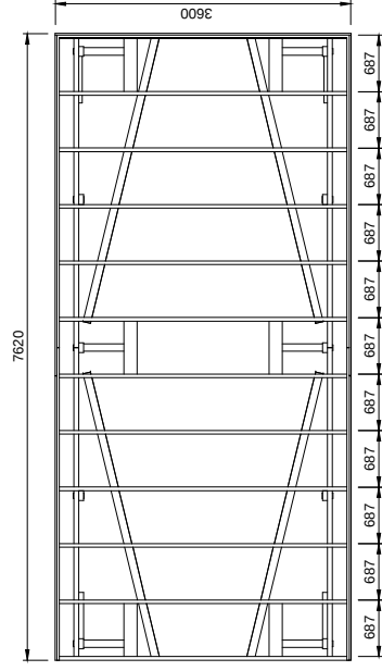
TOP 1:100
